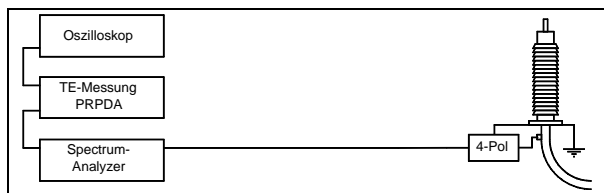
Bild 3 Prinzip der TE-Auskopplung am Kabelschirm
