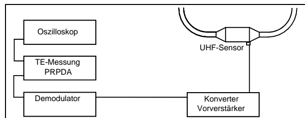
Bild 5 Prinzip der Messung mit Feldsensoren
