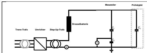
Bild 1 Schema einer Serie-Resonanz-Anlage
