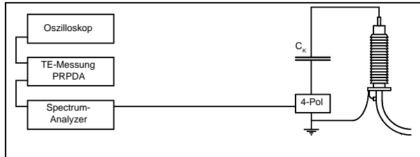
Bild 2 Prinzip der elektrischen TE-Messung mit Koppelkondensator
