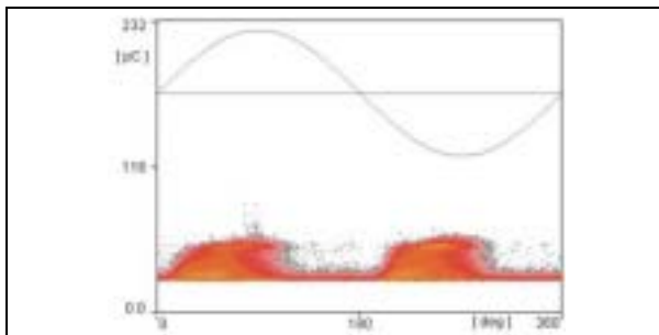
Bild 14 PRPDA-Bild
