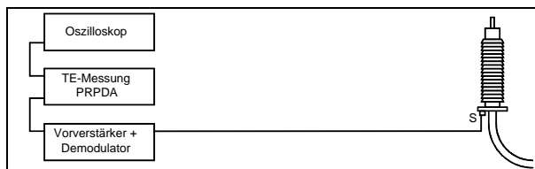
Bild 6 Prinzip der akustischen TE-Messung
