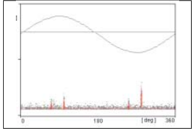
Bild 12 PRPDA-Bild von der dritten Muffe, 1825 m von der Prüfanlage entfernt
