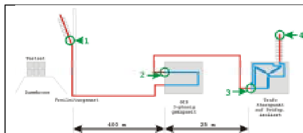
Bild 8 Messprinzip einer integralen Prüfung
