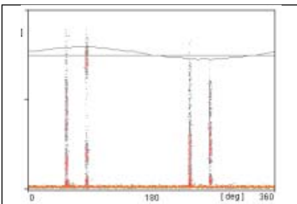
Bild 11 PRPDA-Bild von der ersten Muffe, 396 m von der Prüfanlage entfernt
