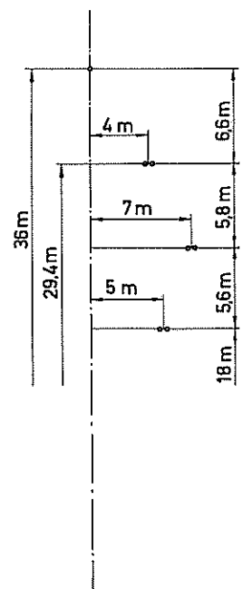
Fig. 2 Leiteranordnung einer 220-kV-Leitung
