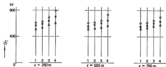
Fig. 17 Wie Fig. 16, aber für eine Stossform des Blitzes von 10/100 \mu s Bezeichnungen siehe Fig. 10
