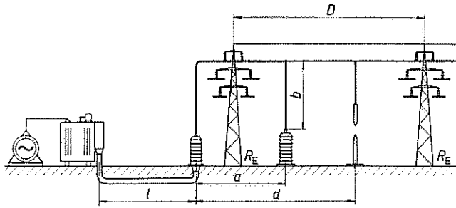
Fig. 1 Disposition der Anlage
