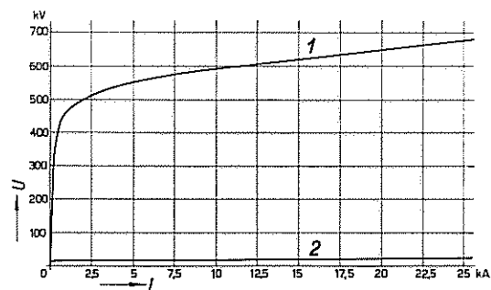
Fig. 4 Ableitercharakteristik (1) und Restspannung der nachgebildeten Funkenstrecke (2)
