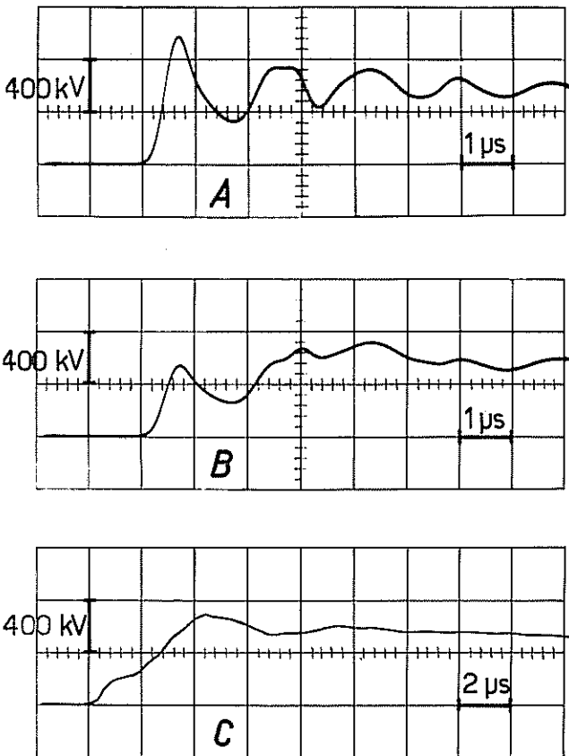
Fig. 15 Spannung am Transformator bei Blitzeseinschlag in den ersten Masten in 250 m Entfernung vom Kabelendverschluss Stärke des Blitzstromes: 100 kA Stossform: 1/100 \mu s Masthöhen: A 40 m, B 20 m, C 0 m Masterdungswiderstand: 10 \Omega Kabellänge: 200 m
