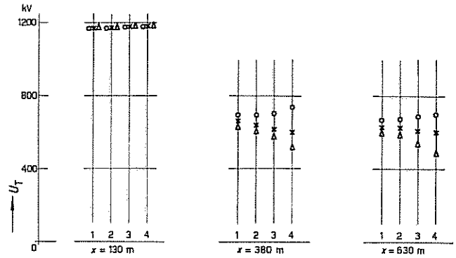
Fig. 16 Transformatorspannung U_T beim Schutz mit Ableiter am Kabelendverschluss in Funktion der Einschlagdistanz x Einschlag in die Mitte der Spannweite Stärke des Blitzstromes: 100 kA Stossform: 2/100 \mu s Kabellängen und Masterdungswiderstände wie in Fig. 10
