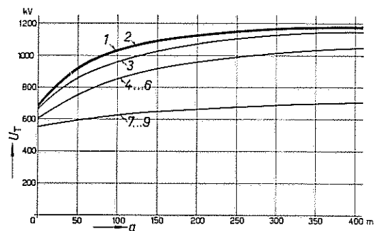
Fig. 5 Transformatorspannung U_T in Funktion der Ableiterdistanz a längs der Freileitung bei weit entferntem Blitzeinschlag Kabellänge 100 m
