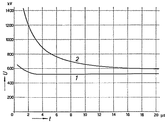
Fig. 3 Ansprechcharakteristik des Ableiters (1) und der Funkenstrecke (2)
