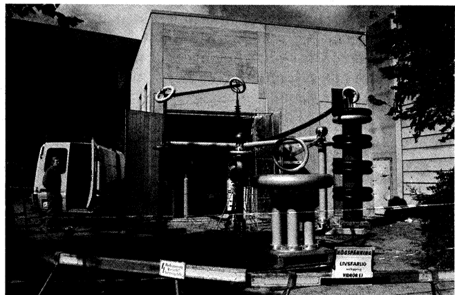
Figur 5 Städtische Unterstation 132 kV, Schweden, im September 1987
