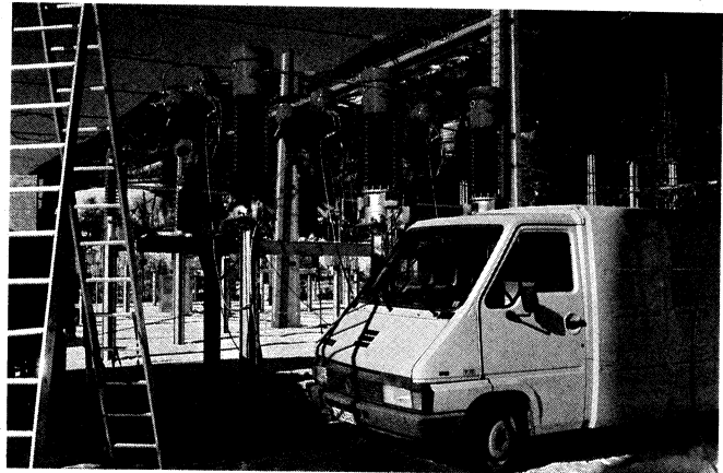
Figur 4 Aussenaufstellung in einer 110-kV-Unterstation, Kärnten, bei den Österreichischen Draukraftwerken (OeDK) im Januar 1988 Brückenschaltung nach Figur 1a
