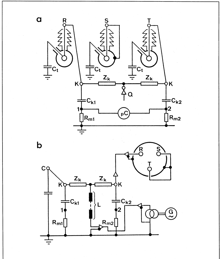
Figur 2 Doppel-Straight-Schaltung mit Hocheinspeisung durch Resonanz-Stromquellen, Beispiele für TE-Messung an SF 6 -Anlagen
